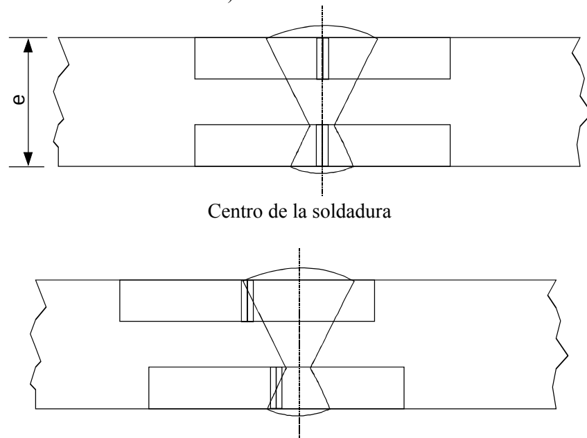
Zona de alteración debida a la soldadura
