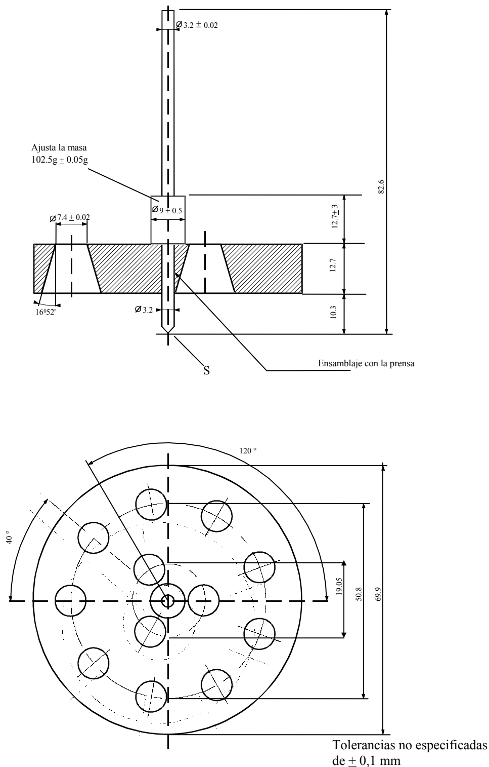
Figura 1 - Penetrómetro
